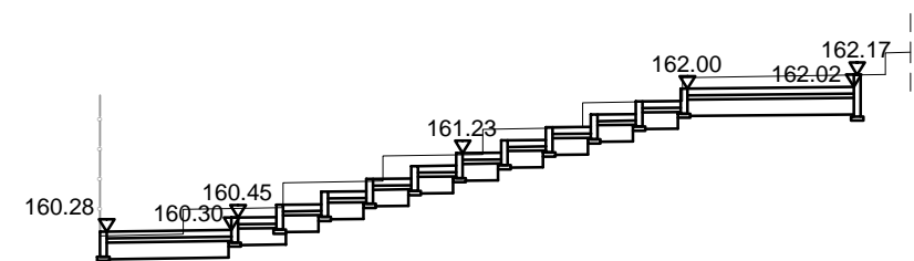
Przekrój 6-6
