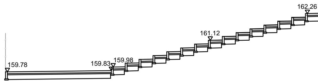
Przekrój 1-1
