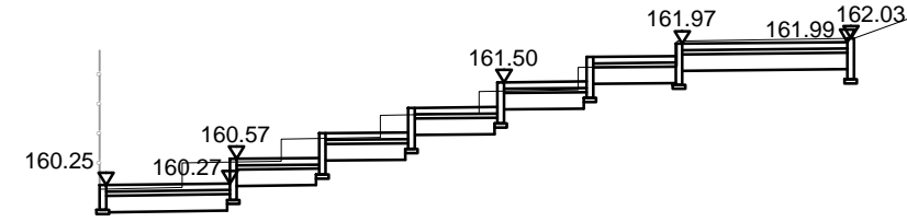
Przekrój 5-5
