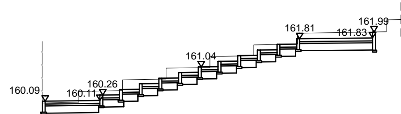
Przekrój 2-2
