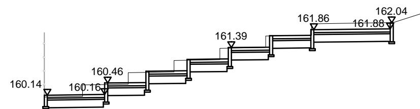
Przekrój 3-3
