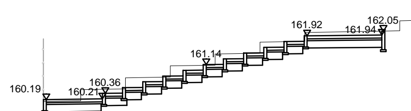
Przekrój 4-4
