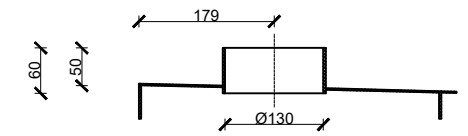
Szczegół A
